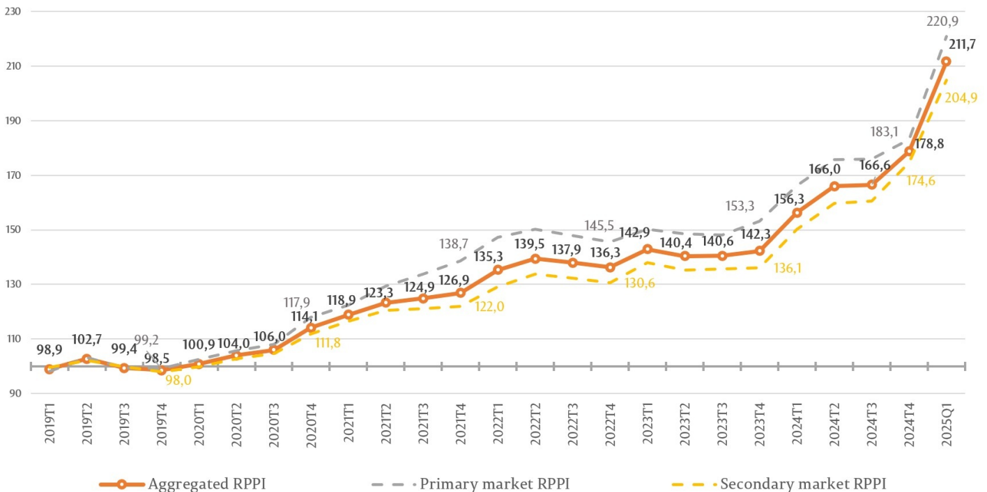
Figure 1. RPPI, % (average_2019=100)
